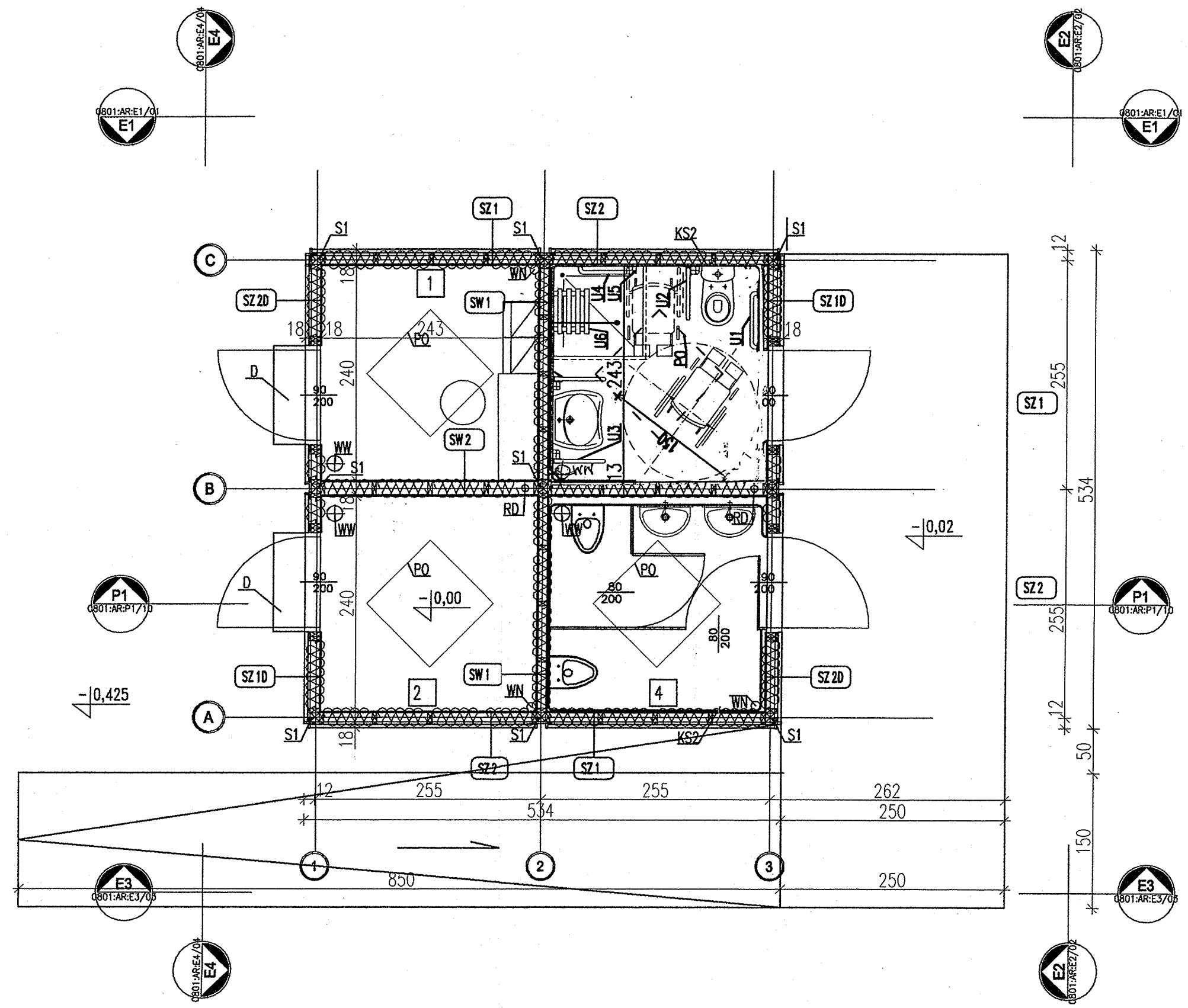
RZUT PRZYZIEMIA 1:50
