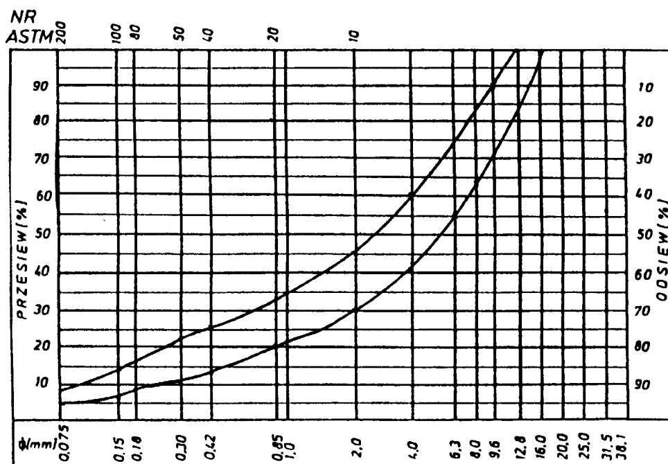
Rys. 13. Krzywe graniczne uziarnienia mieszanki mineralnej 0 □ 16 mm do warstwy wiążącej, z betonu asfaltowego dla KR 4
