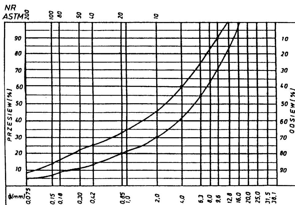
Rys. 13. Krzywe graniczne uziarnienia mieszanki mineralnej 0+12,8 mm do warstwy z betonu asfaltowego dla KR 1
